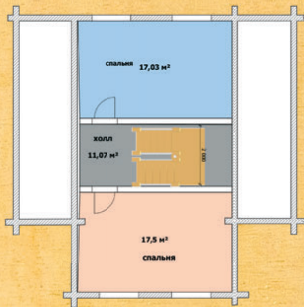
План мансардного этажа
